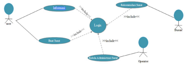
Gambar 4. Usecase interaksi antara sistem dan aktor
